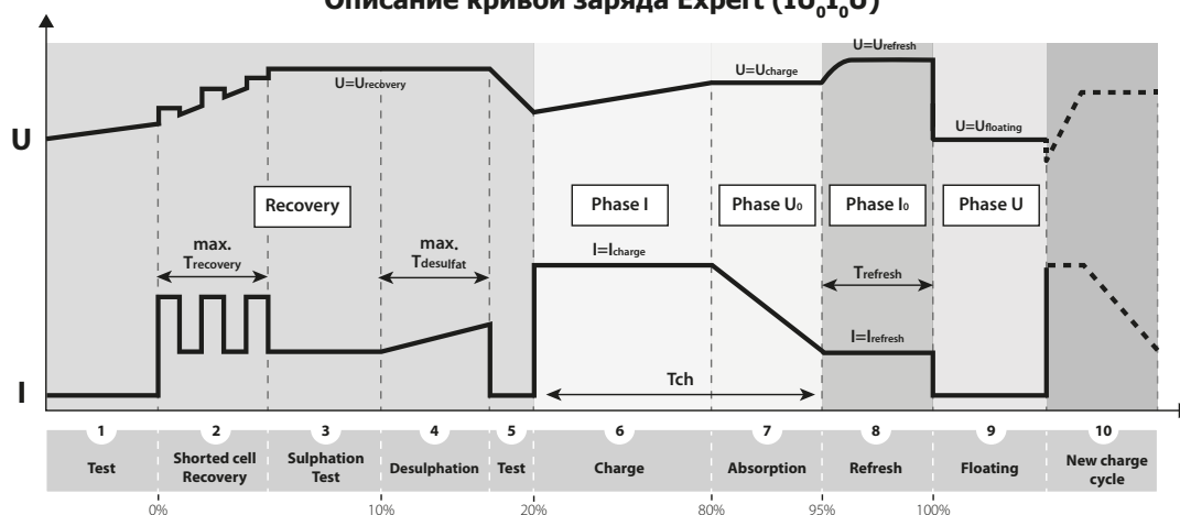
Описание кривой заряда Expert ( I U_0 I_0 U )
